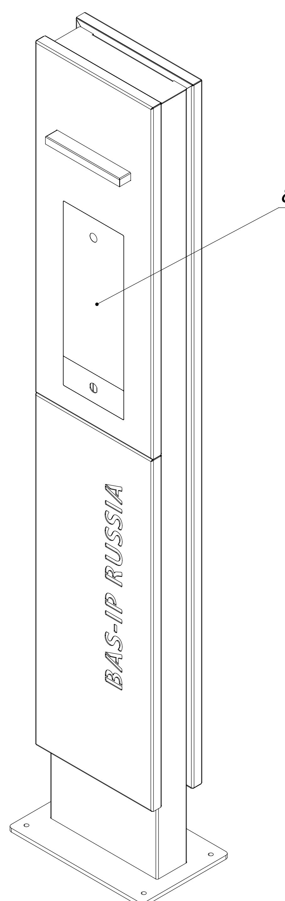
Стойка с панелью AA-14FB
