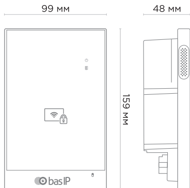
Вызывная панель
