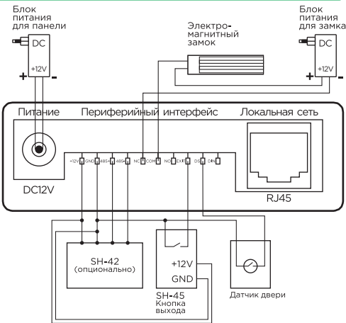
Схема подключения электромагнитного замка с использованием внешнего блока питания для замка.
